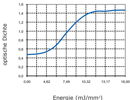
Dynamische Sensitivität
