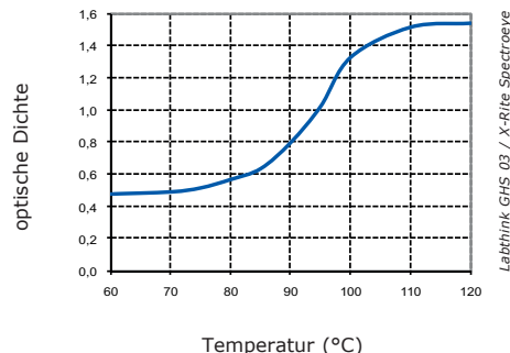
Statische Sensitivität
